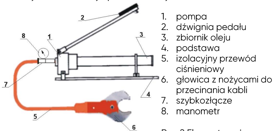
Rys. 2 Elementy nożyc
