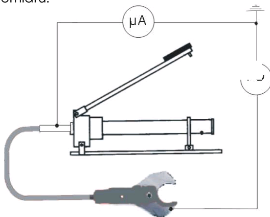
Rys. 4 Układ do badania wytrzymałości i pomiaru prądu upływu
